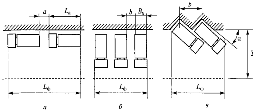
Рис. .1. Схемы для расчета площадки для маневрирования при различных способах расстановки автотранспортного средства: а — поточная (боковая); б — торцевая; в — ступенчатая
