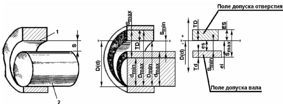
Рисунок 3. Посадка с зазором
