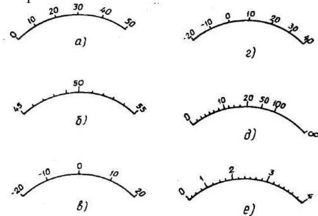
Рисунок 1 - Виды шкал СИ
