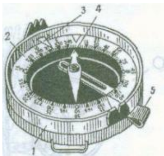
Рис. Компас Адрианова: 1 — крышка со стойками для визирования; 2 — лимб; 3 — указатель отсчета; 4 — магнитная стрелка; 5 — тормоз.
