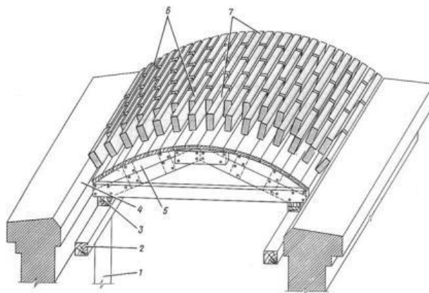
Рис Кладка сводов: 1 – стойка; 2 – горизонтальный брус, поддерживающий опалубку; 3 – клинья; 4 – пята; 5 – кружальная опалубка;
