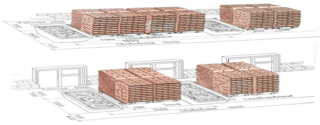
Рис. 1 Рабочее место каменщика при кладке стен
