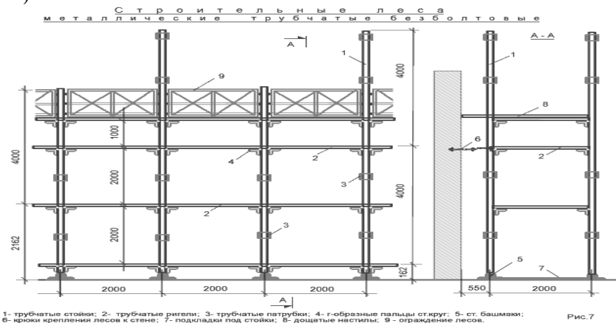
Рис.3 Строительные леса металлические трубчатые безболтовые
