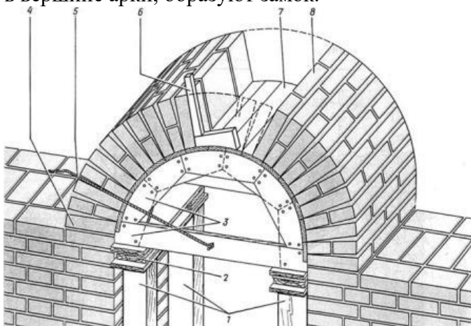
Рис. Кладка арочной перемычки: 1 – стойки, поддерживающие опалубку;
