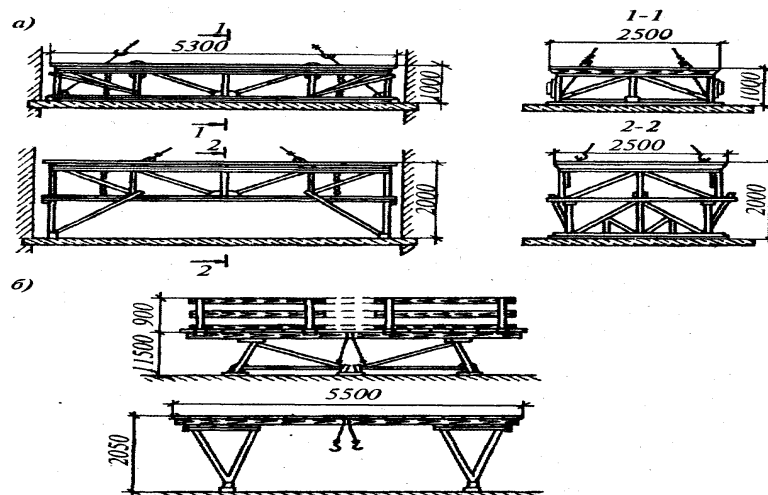
Рис.2 Подмости для каменной кладки
