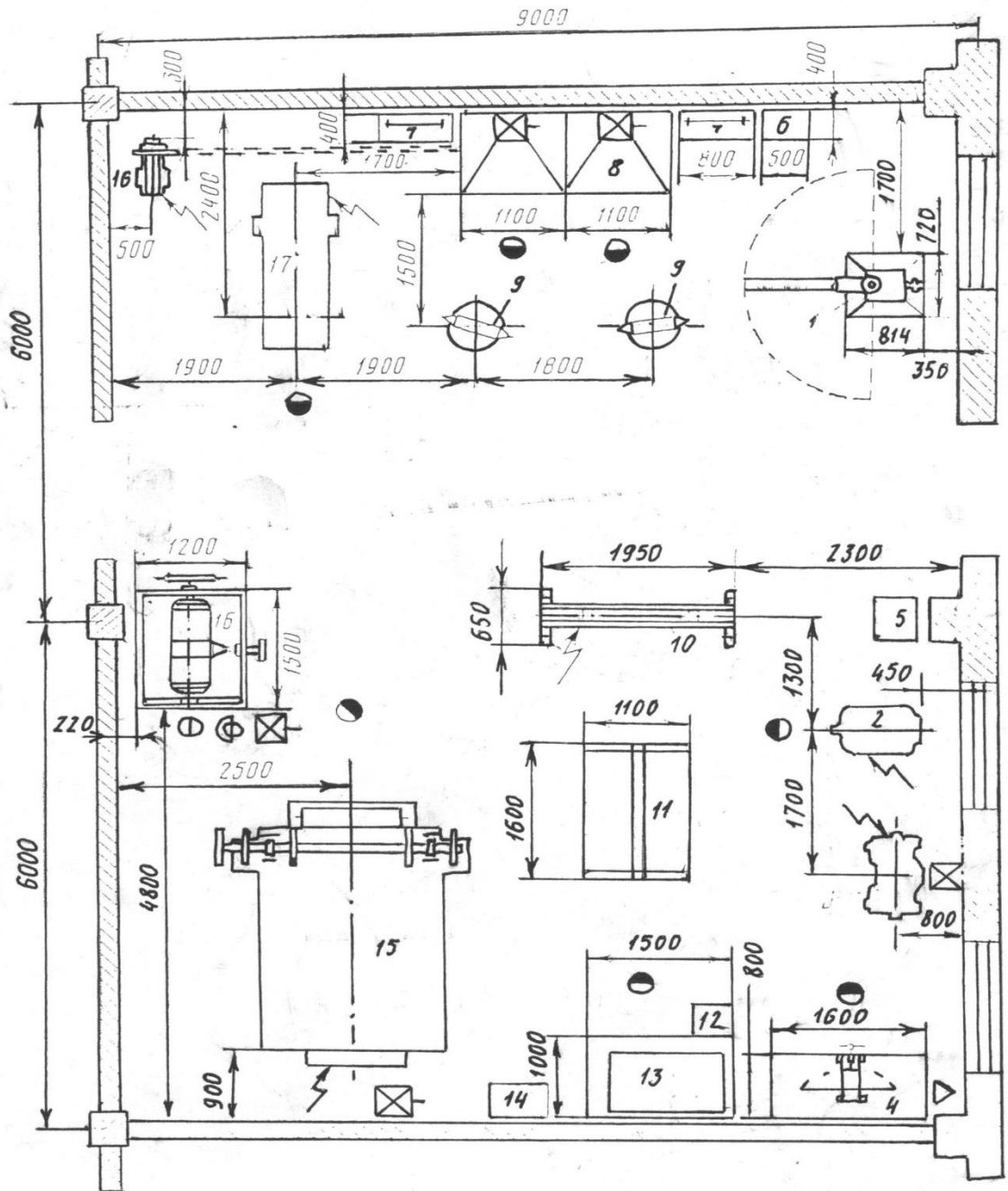
Планировка кузнечно-рессорного отделения:
