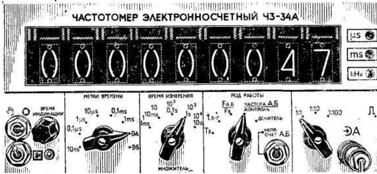
Рисунок 4 - Лицевая панель частотомера класса точности 2,0 с номинальной частотой 50 Гц и равномерной шкалой
