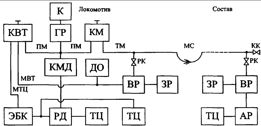
Рис. 4.1. Структурная схема тормозного оборудования грузовых поездов
