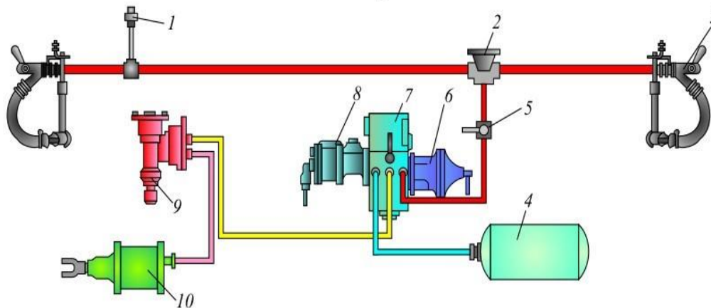
Схема тормозного оборудования грузового вагона с воздухораспределителем №270-005-1 или 483 и авторежимом 265А-000
