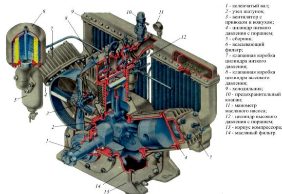
Схема компрессоров КТ6, КТ7, КТ6Эл
