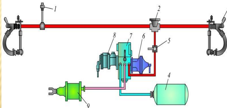
Схема тормозного оборудования грузового вагона с воздухораспределителем №270-005-1 или 483
