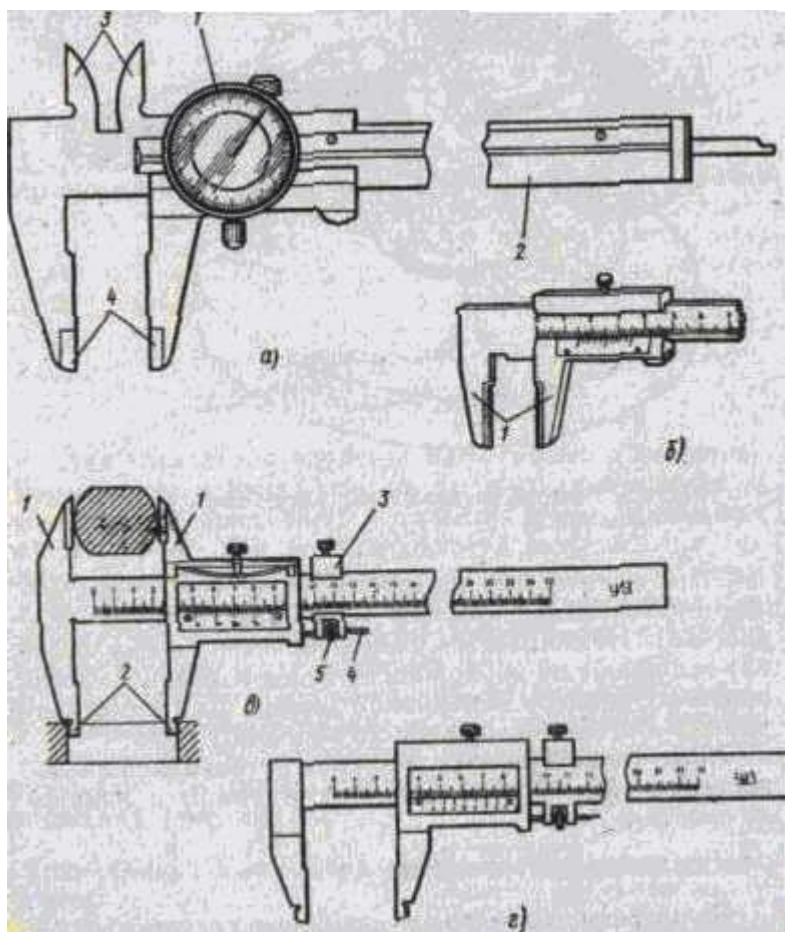
Рисунок 1 - . Штангенциркули: а - ШЦ-1С; б - ШЦТ-1; в - ШЦ-П; г – ШЦ-Ш.
