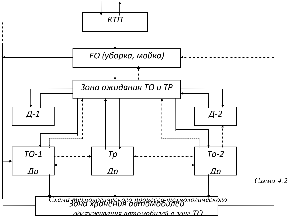
Схема технологического процесса ТО и ремонта автомобилей на АТП
