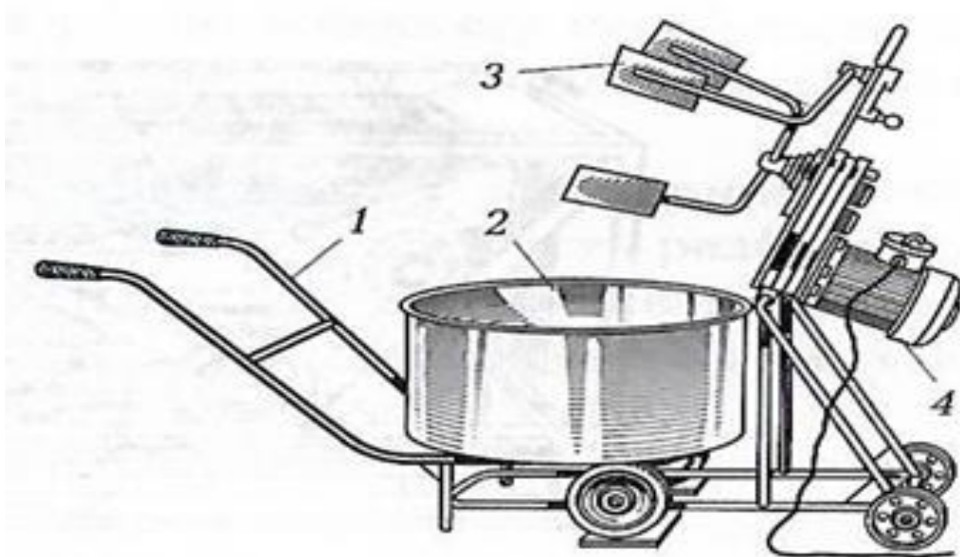
Рис. 5.2. Растворосмеситель: СО-23В:
