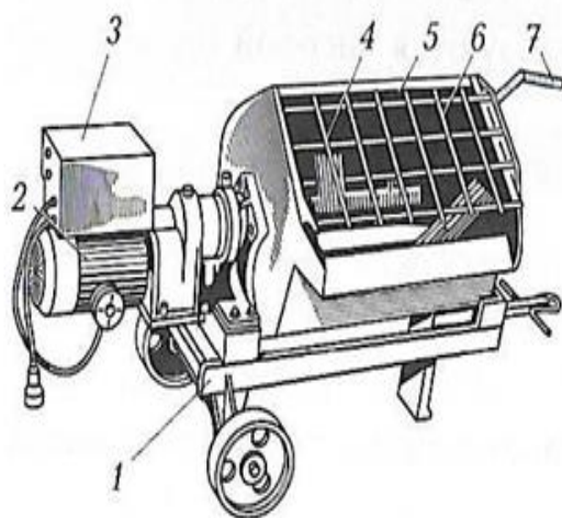
Рис. 5.1. Растворосмеситель: СО-46Б:
