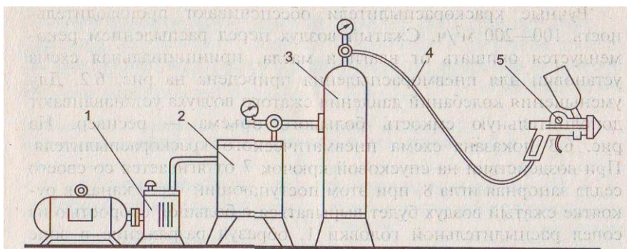
Рис. 6.2. Схема установки для пневматического распыления: 1 — компрессор; 2 — маслоуловитель; 3 — ресивер; 4 — гибкий шланг; 5 — краскораспылитель
