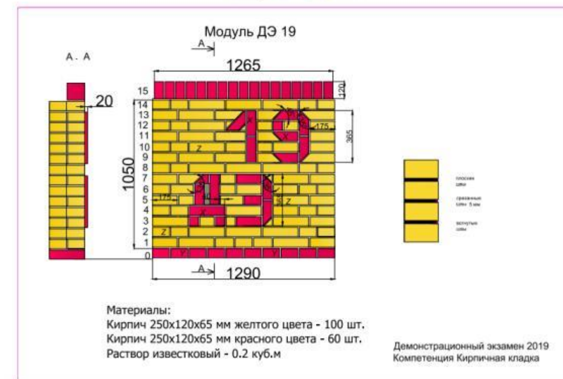
Рисунок. Пример схемы модуля
