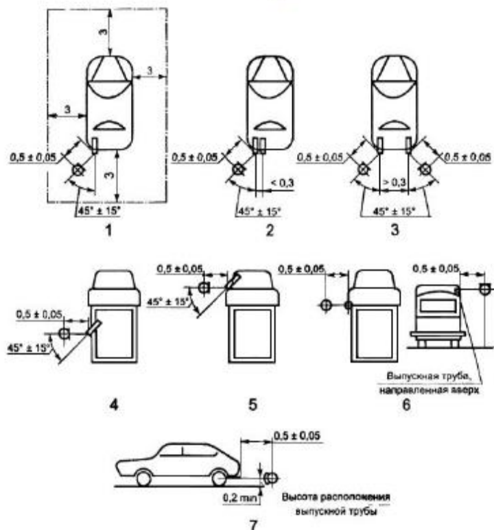
Рисунок 1 - Схемы установки микрофонов при различном расположении выпускных труб. 1-5 - установка микрофонов относительно выпускной трубы в горизонтальной плоскости; 6 - установка микрофонов относительно вертикально расположенной выпускной трубы; 7 - установка микрофонов относительно выпускной трубы в вертикальной плоскости.
